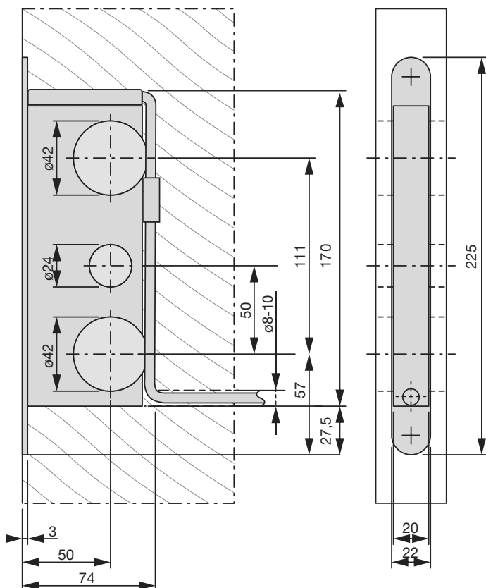
Urtagsritning Protector 9197 och Protector HD 9197
